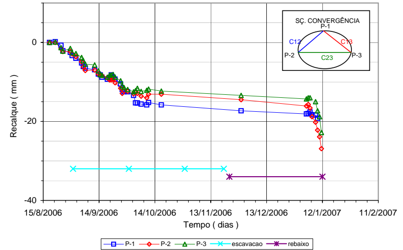
BUREAU DE PROJETO E CONS. LTDA. METRO LINHA 4 - TRECHO PINHEIROS Recalque - SEÇÃO 7.0+86,65 - SENTIDO FERREIRA DE ARAÚJO
