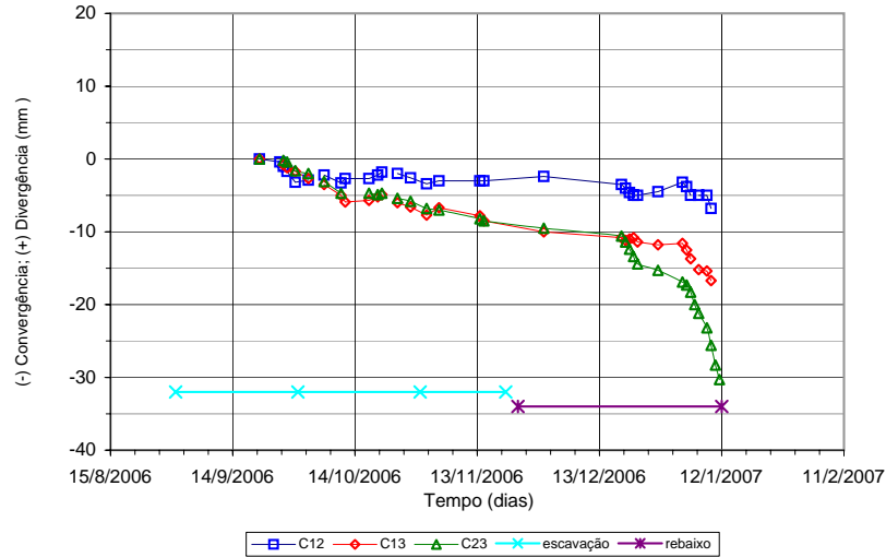
BUREAU DE PROJETO E CONS. LTDA. METRO LINHA 4 - TRECHO PINHEIROS Convergência - SEÇÃO 7.0+96,85 - SENTIDO FARIA LIMA
