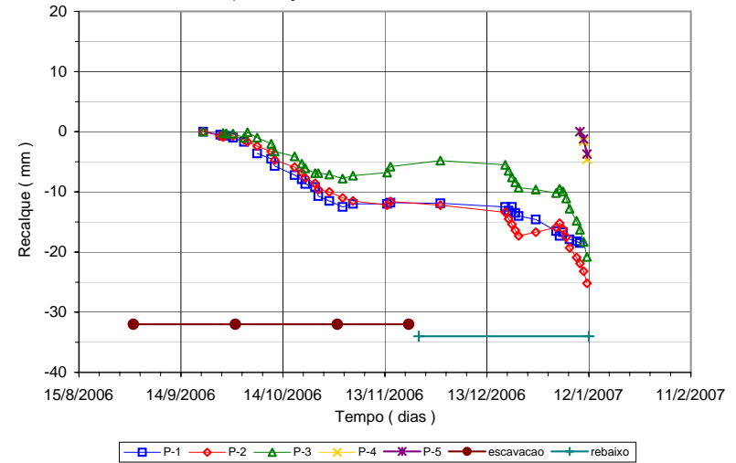
BUREAU DE PROJETO E CONS. LTDA. METRO LINHA 4 - TRECHO PINHEIROS Recalque - SEÇÃO 7.0+96,85 - SENTIDO FARIA LIMA
