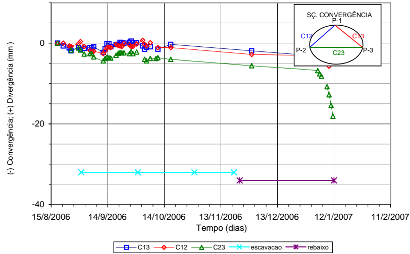
BUREAU DE PROJETO E CONS. LTDA. METRO LINHA 4 - TRECHO PINHEIROS Convergência - SEÇÃO 7.0+86,65 - SENTIDO FERREIRA DE ARAÚJO
