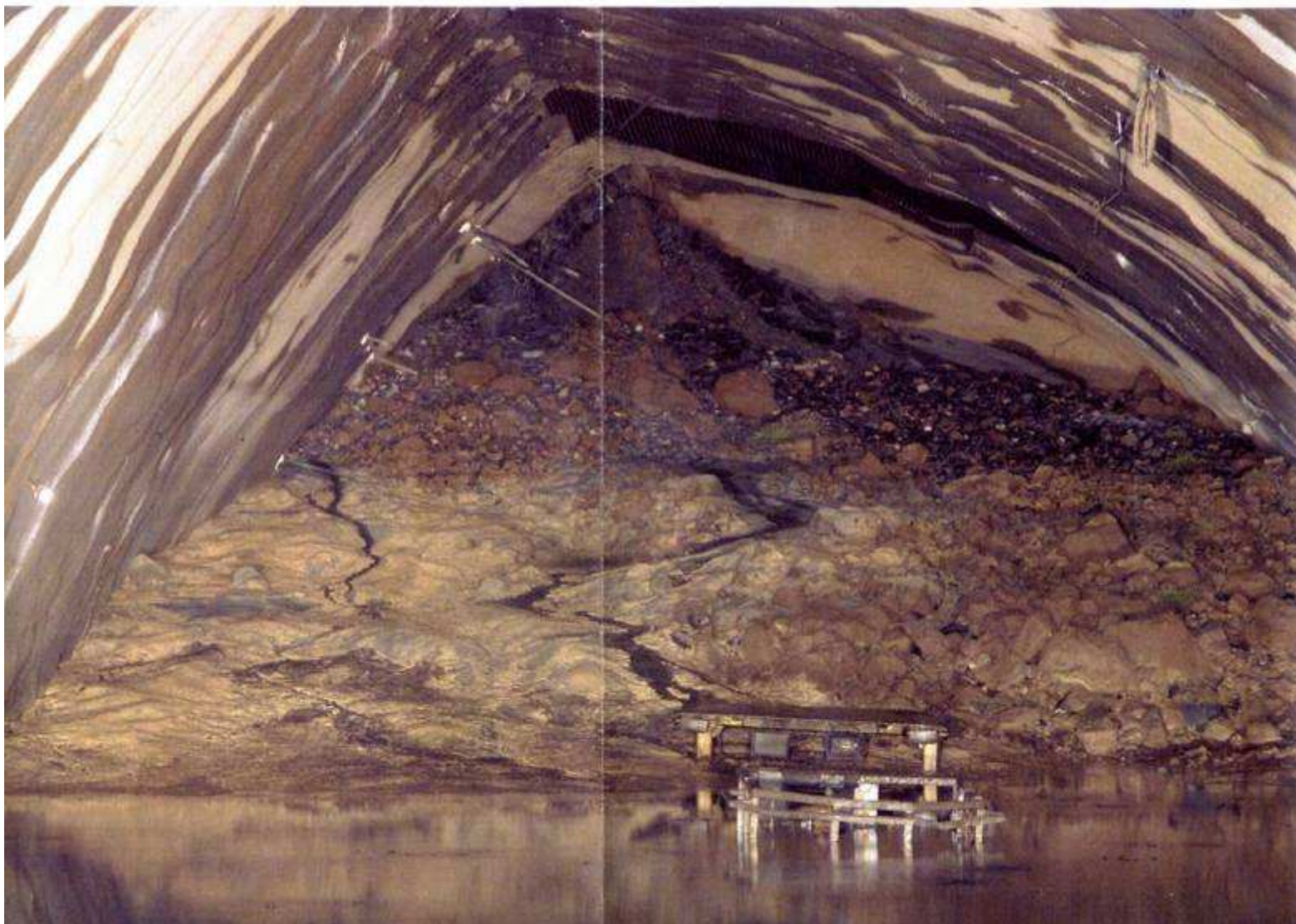
Pohled na čelbu u druhého propadu z prostoru severní tunelové trouby Blanka
