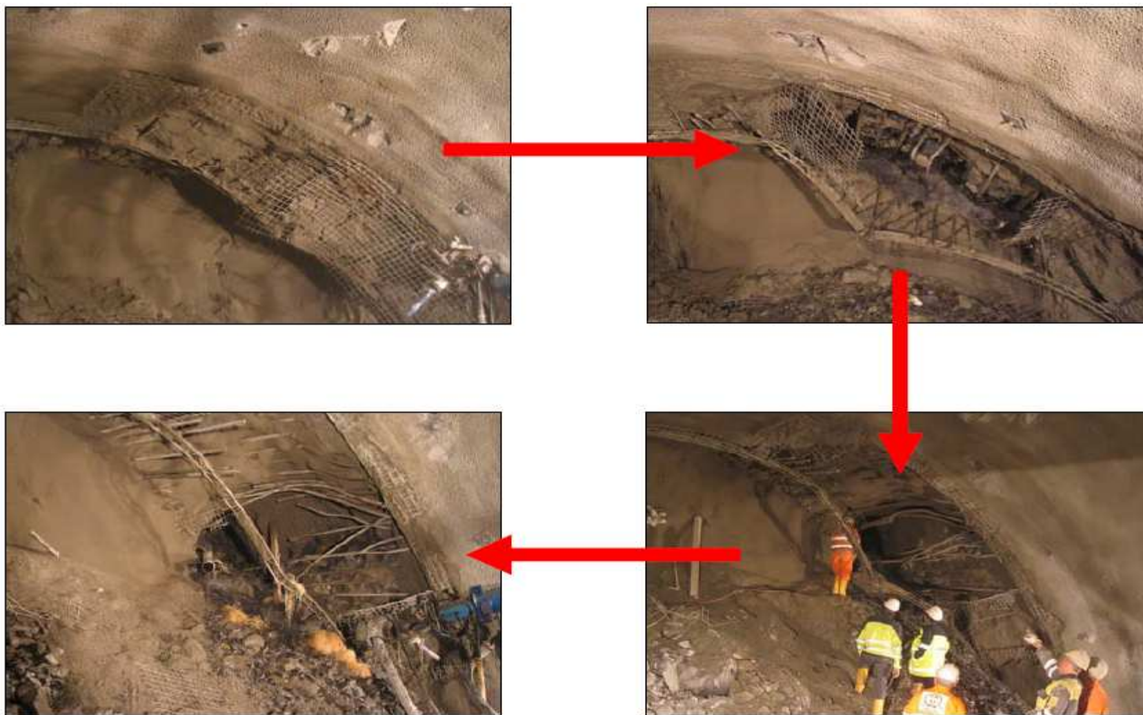
Průběh havárie opěrové části ostění, která vyvrcholila průvalem podzemní vody –tunel Wienervald 2005
